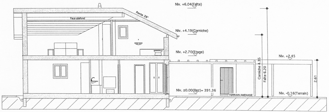
coupe
